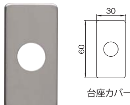
台座カバー
