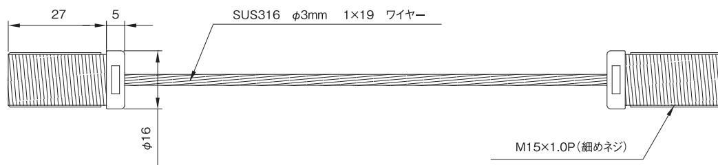
スクエアタイプ 使用ワイヤー径 3mm ※台座四角形
