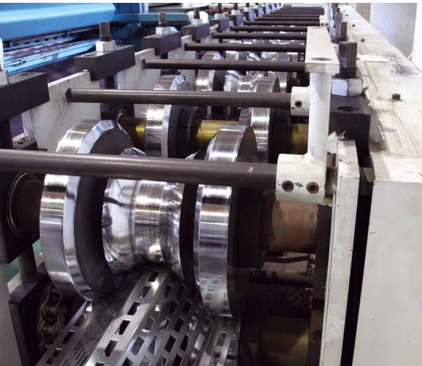
ロールフォーミング成形機による曲げ加工
