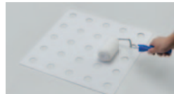
墨出した後にゲージを固定し、ゲージの上からプライマー塗布
