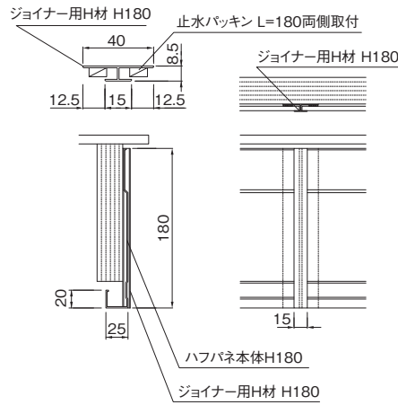
ジョイナー用H材 H180 納まり図
