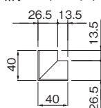
出隅コーナーキャップ
