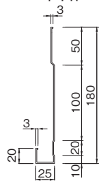
ハフパネ2段用
