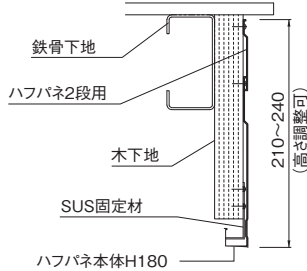
2段納まり図 (鉄骨下地)
