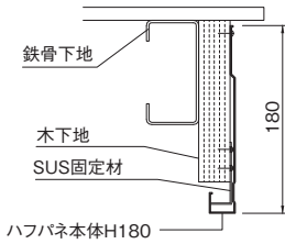
1段納まり図 (鉄骨下地)
