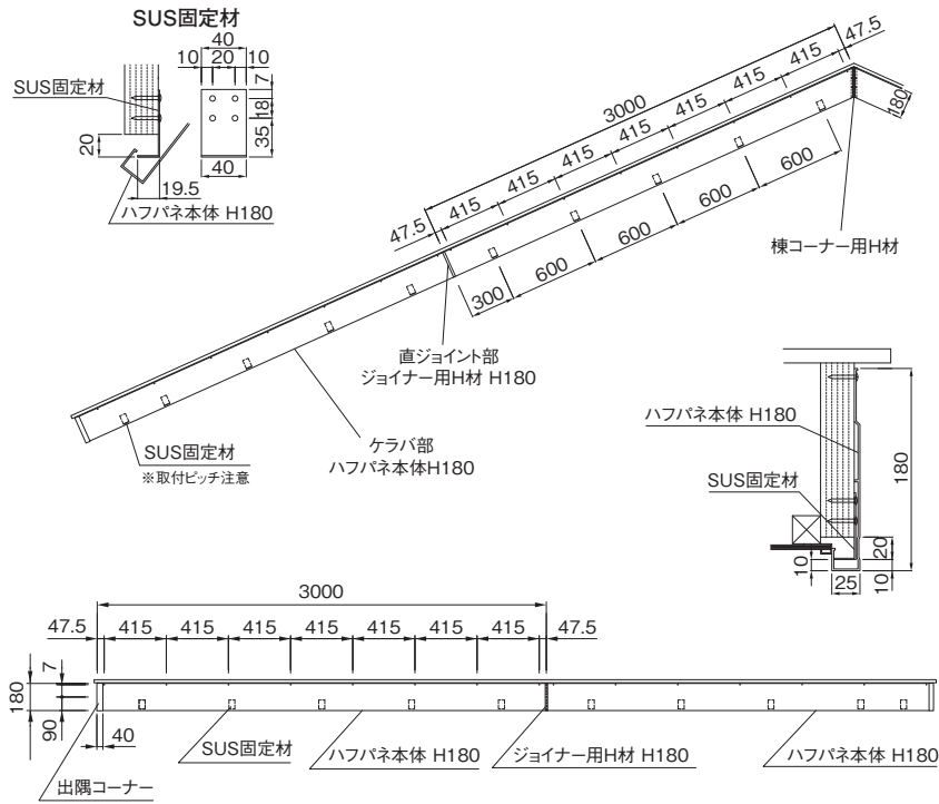
1段納まり図 (鉄骨下地)
